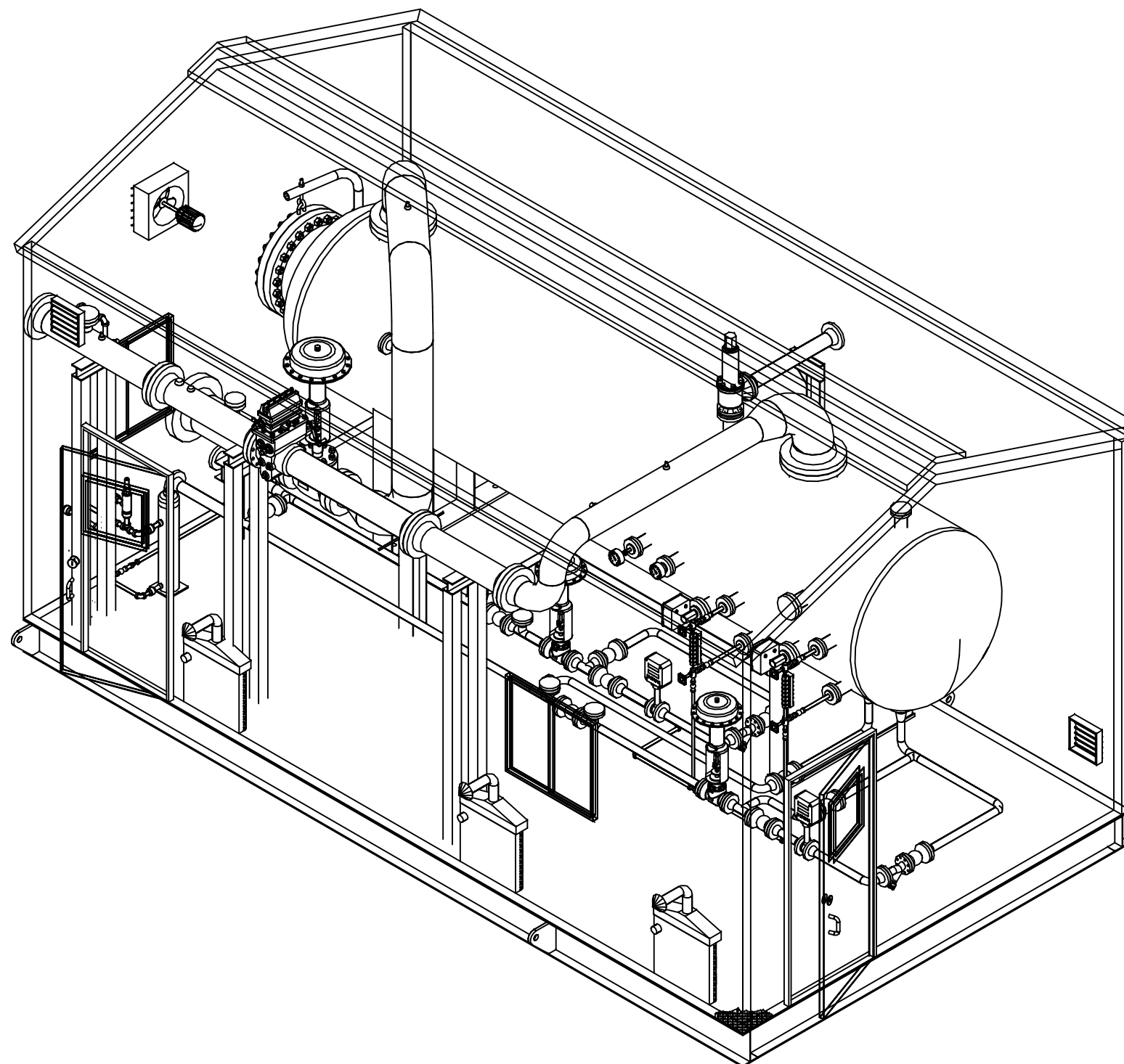
SE ISOMETRIC
